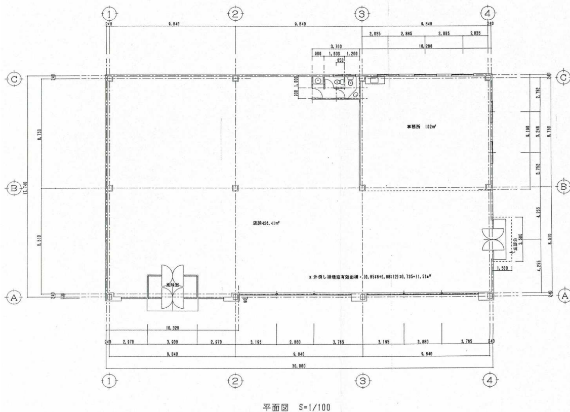
建物平面図等
