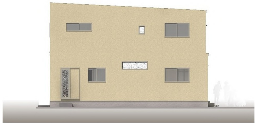
西面立面図 S=1/100
