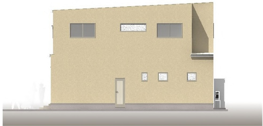
東面立面図 S=1/100
